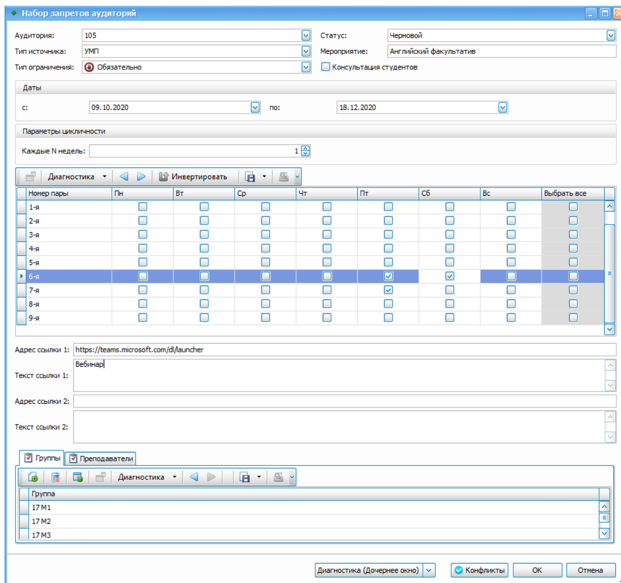
Рис. 42. Запрет аудитории по парам
