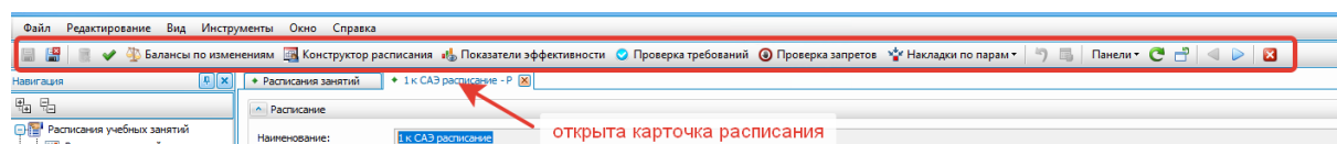
Рис. 50. Панель инструментов окна редактирования карточки расписания
