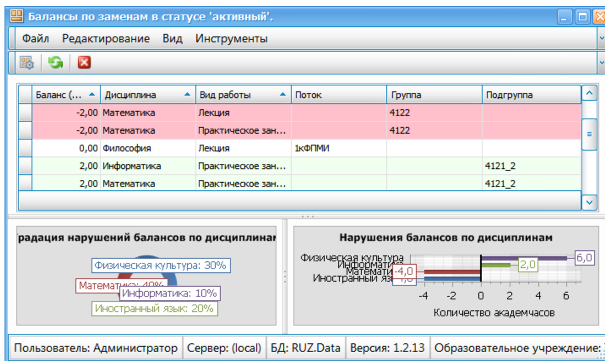
Рис. 51. Балансы по заменам
