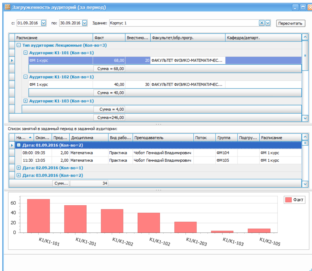
Рис. 47. Загруженность аудиторий за период (сводная информация)
