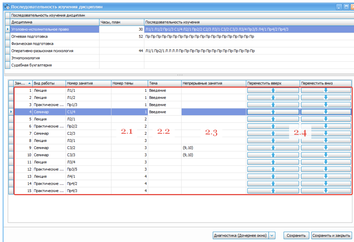
Рис. 40. Окно создания последовательности изучения дисциплины
